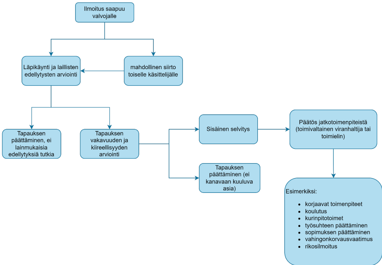
Kuva 1 Ilmoituksen käsittelyprosessi
